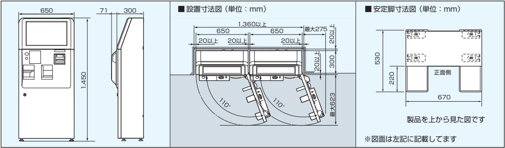
VT-G21シリーズ 寸法図（単位：mm）
