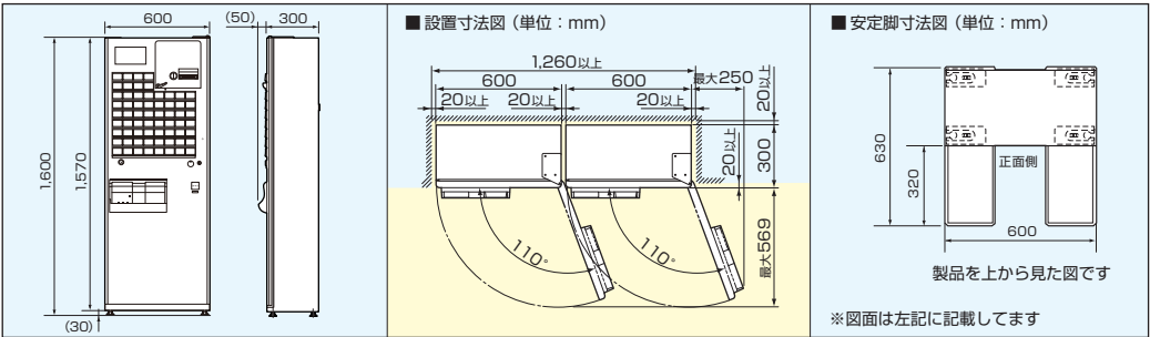
VT-B20シリーズ 寸法図（単位：mm）
