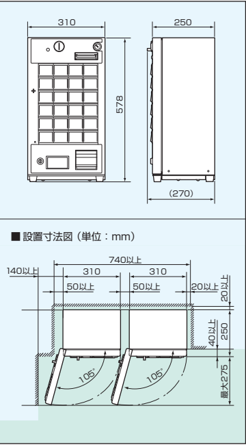
VT-S20シリーズ 寸法図（単位：mm）
